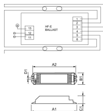
Scheda tecnica Philips Essential HF-E Sfericaast 1/2 55-58 W per TL5 - TL-D
